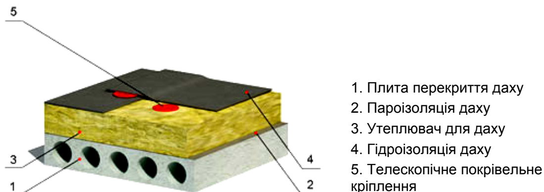
Рисунок 7.1.6. Структура утеплення дахового перекриття
